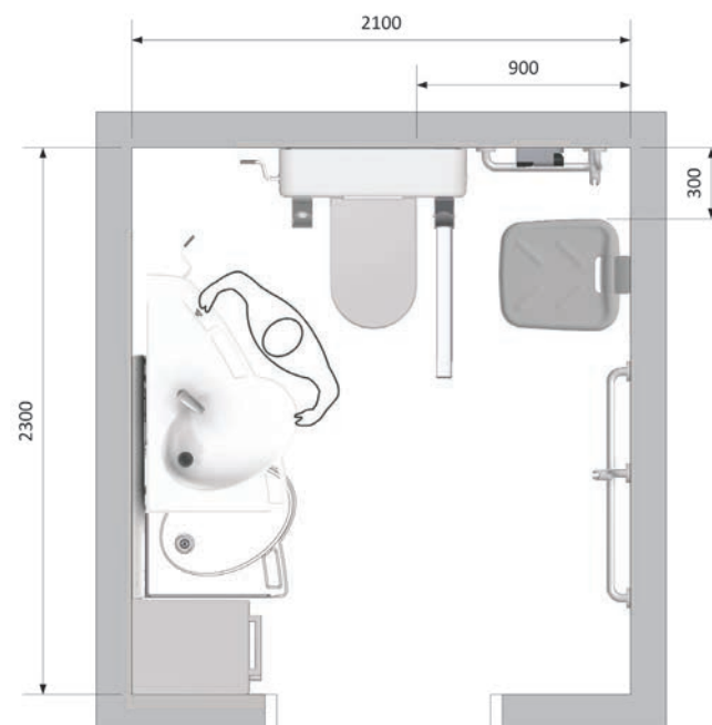
Baño para usuarios con dificultades para caminar
