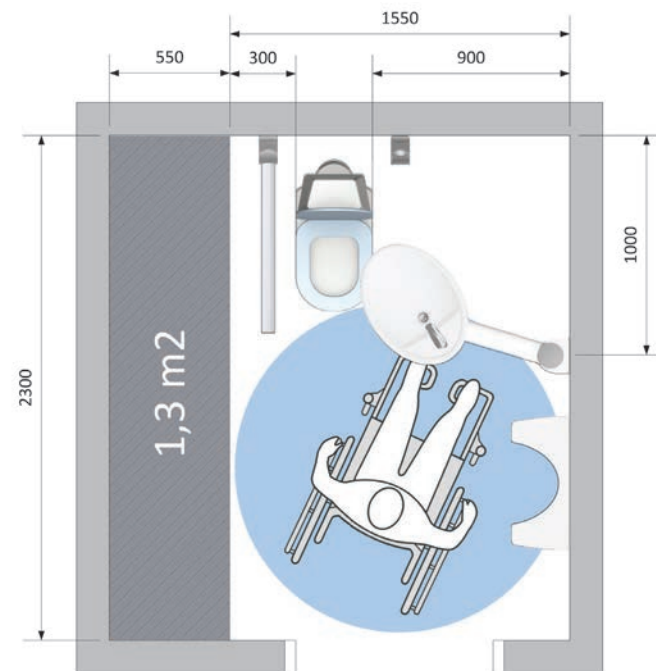
Baño para usuarios autosuficientes de sillas de ruedas El área del baño se puede reducir en 1,3 m² en comparación con un baño estándar.
