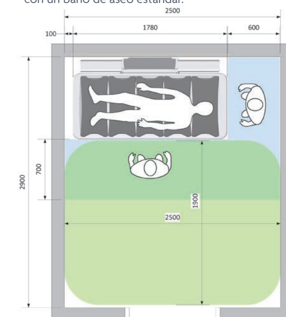
Ducha / cambiador para usuarios que necesitan la asistencia de un cuidador en instituciones
