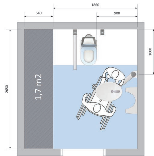
Baño para usuarios de sillas de ruedas que necesitan la ayuda de un cuidador El área del baño se puede reducir en 1,7 m² en comparación con un baño de aseo estándar.
